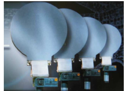
FLIZ-Schweißspiegel HG 200 T 230 V 800 Watt mit Koffer Eugen Riexinger GmbH_Co.KG
